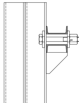
Knaggen zur Übertragung von Längskräften appets for the longitudinal forces
